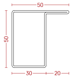
MF 5030L Z
