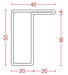
MF 5020L D MF 5020L Z
