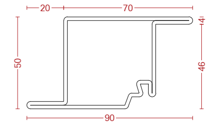
MF 5050ZG D MF 5050ZG Z
