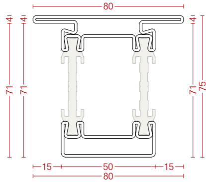
FT 7550TF-02 FT 7550TF-05 FT 7550TF-07 FT 7550TF-12
